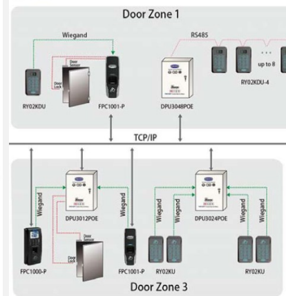
系统图
