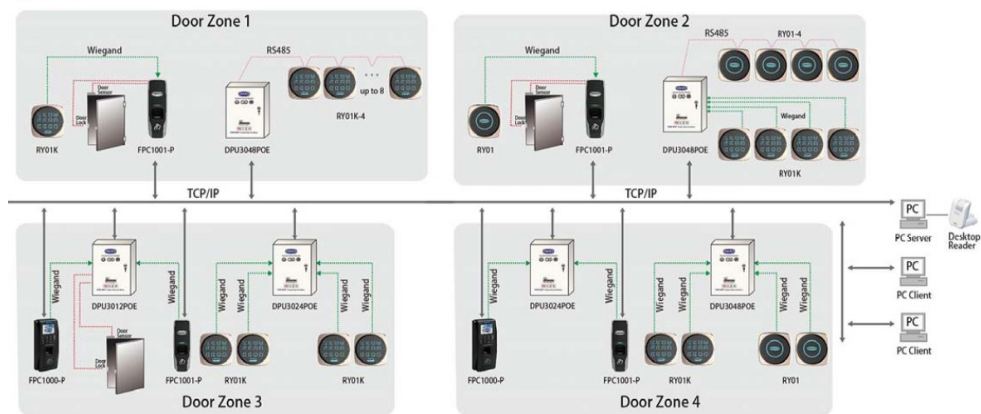
系统图
